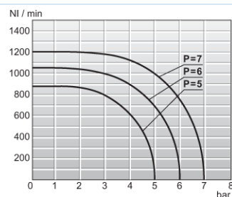
Průtokový diagramm 1/8"
