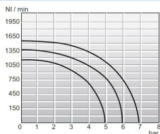
Průtokový diagramm 1/4"
