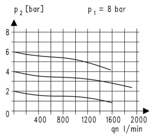
Průtokový diagram
