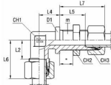
s řezným kroužkem B4
