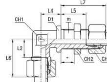
s řezným kroužkem B3
