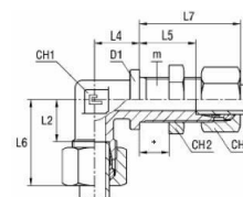
mit B3-Schneidring
