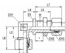
mit B4-Schneidring
