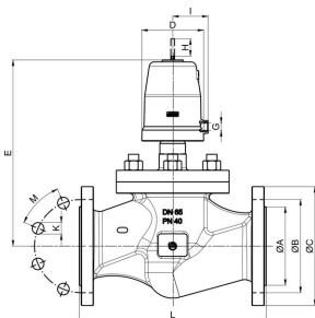
Sprężyna zamyka, Typ SE24, SE25, SE33
