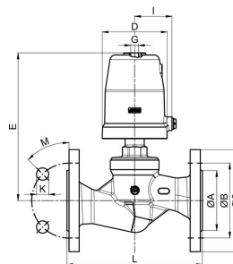
Sprężyna otwiera, Typ SE23
