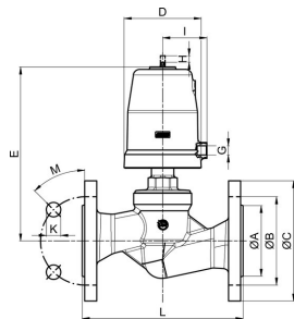
Sprężyna zamyka, Typ SE24, SE25, SE33
