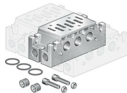
Center piece Typ BMI2
