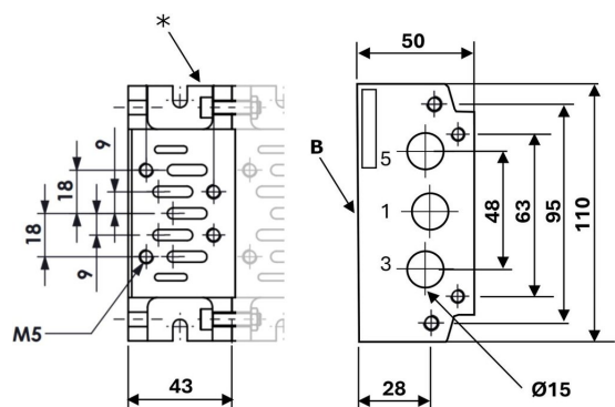
Center piece type SBI1-CE
