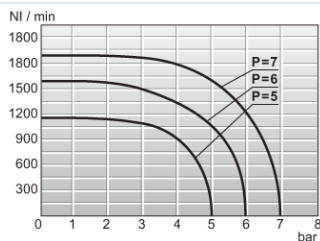
Virtauskaavio 1/4"
