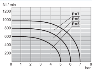
Virtauskaavio 1/8"
