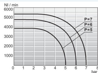
Virtauskaavio 1/2"
