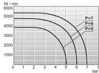
Diagramma di portata 1/2"
