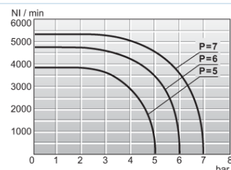
Strømningsdiagramm 1/2"
