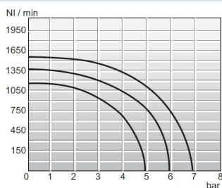
Virtauskaavio 1/4"
