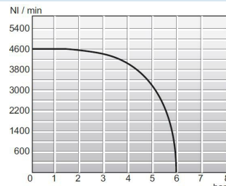
Strømningsdiagramm 1/2"
