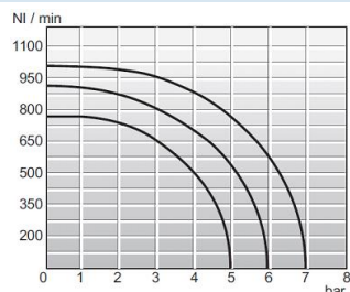
Strømningsdiagramm 1/8"
