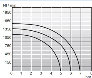
Doorstroomdiagramma 1/4"
