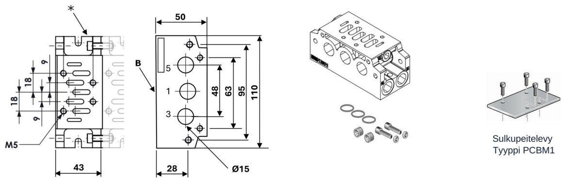
Välikappale tyyppi SBI1-CE
