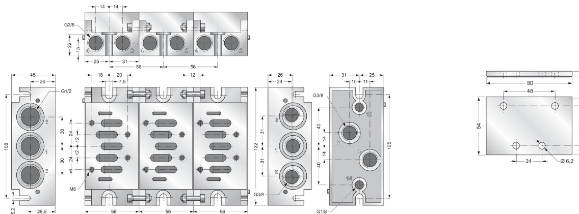
Välikappale Typ BMI2
