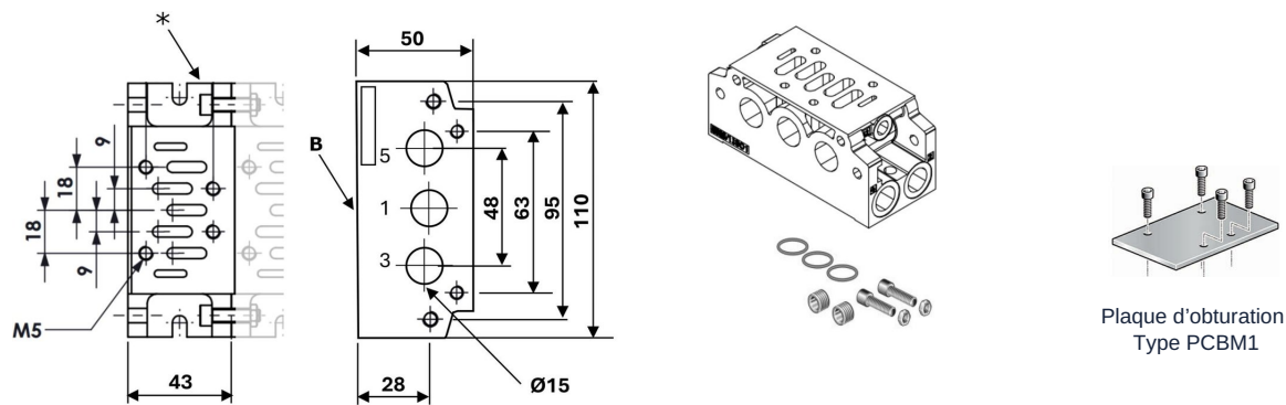
Pièce intermédiaire type SBI1-CE
