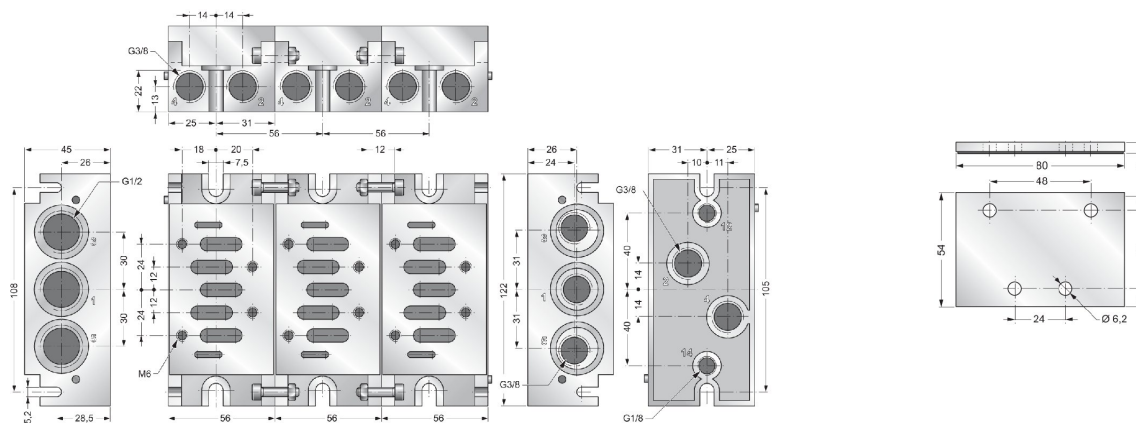
Raccord de connexion Typ BT12
