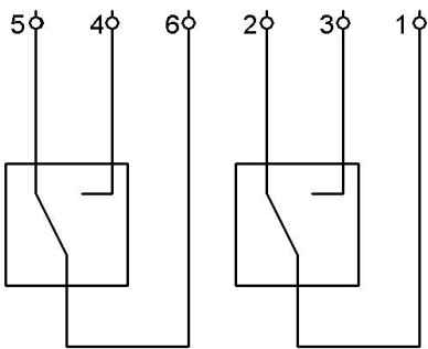
Señales de fin de carrera: 1-2-3...CERRADO 4-5-6...ENCENDIDO
