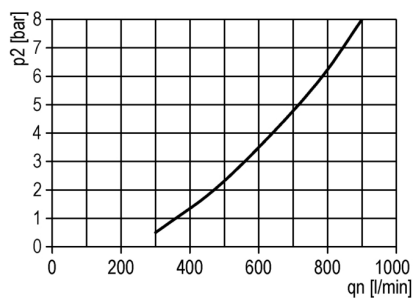
Olievernevelaar-inschakeldrempel
