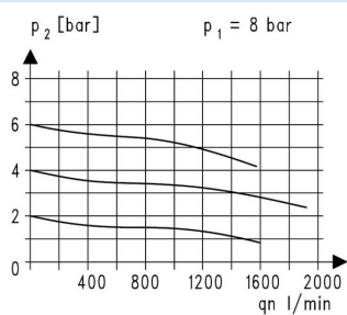
Diagramă de debit
