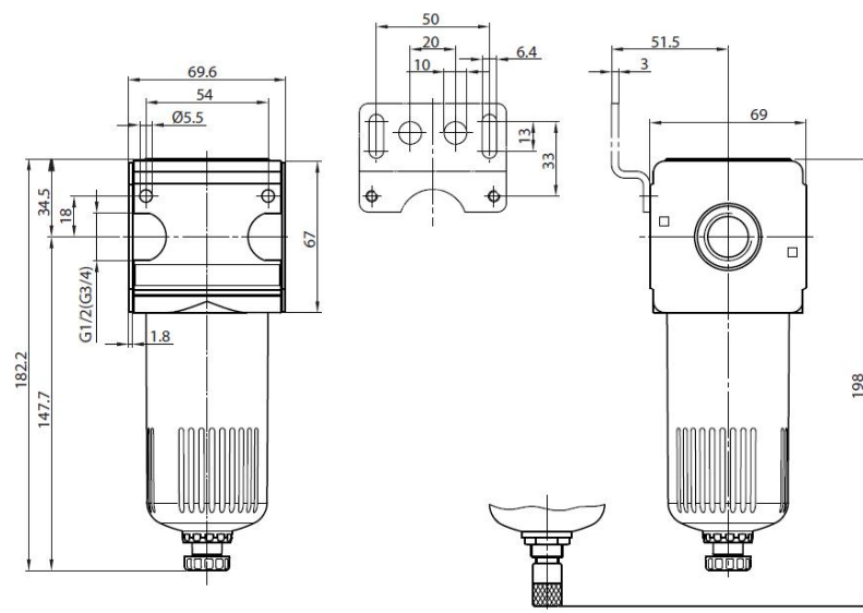
automatisk aftapningsventil
