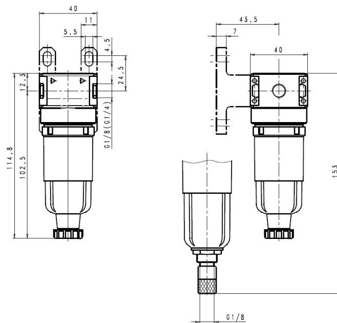
automatiskt avtappningsventil
