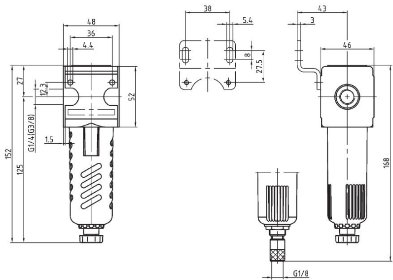
automatisch aftapventiel
