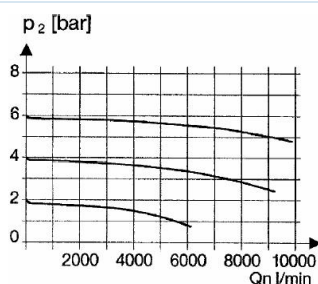
Strømningsdiagram
