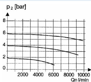
Strømningsdiagramm
