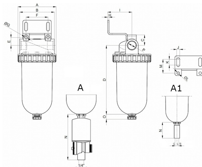
A, A1: automatiskt avtappningsventil
