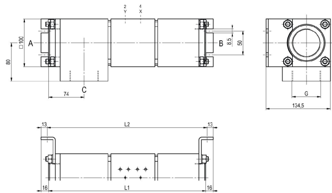
CVTV3-50 Funktion NC
